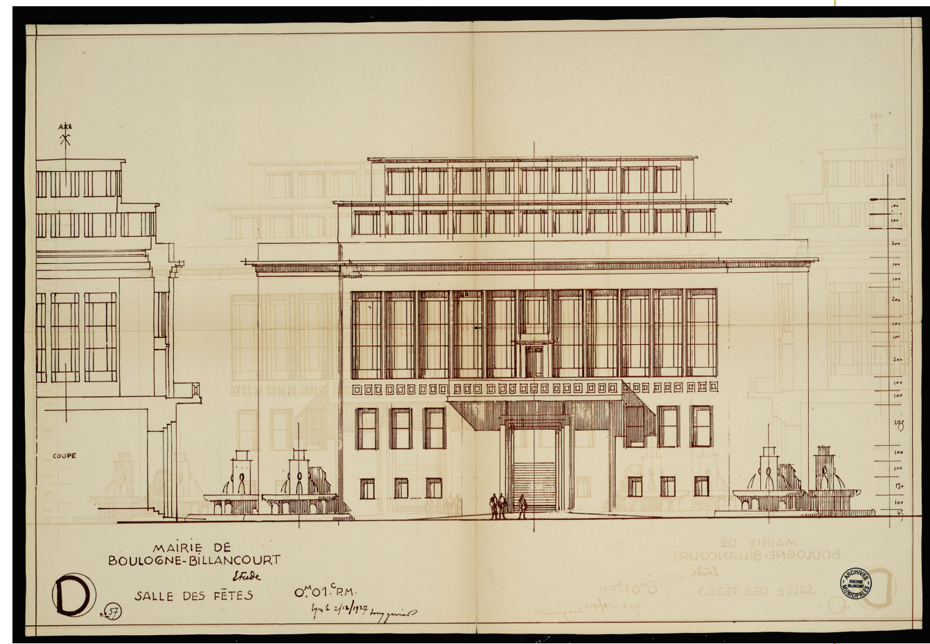
Projet de façade 2 décembre 1927 - 1 M1 57
