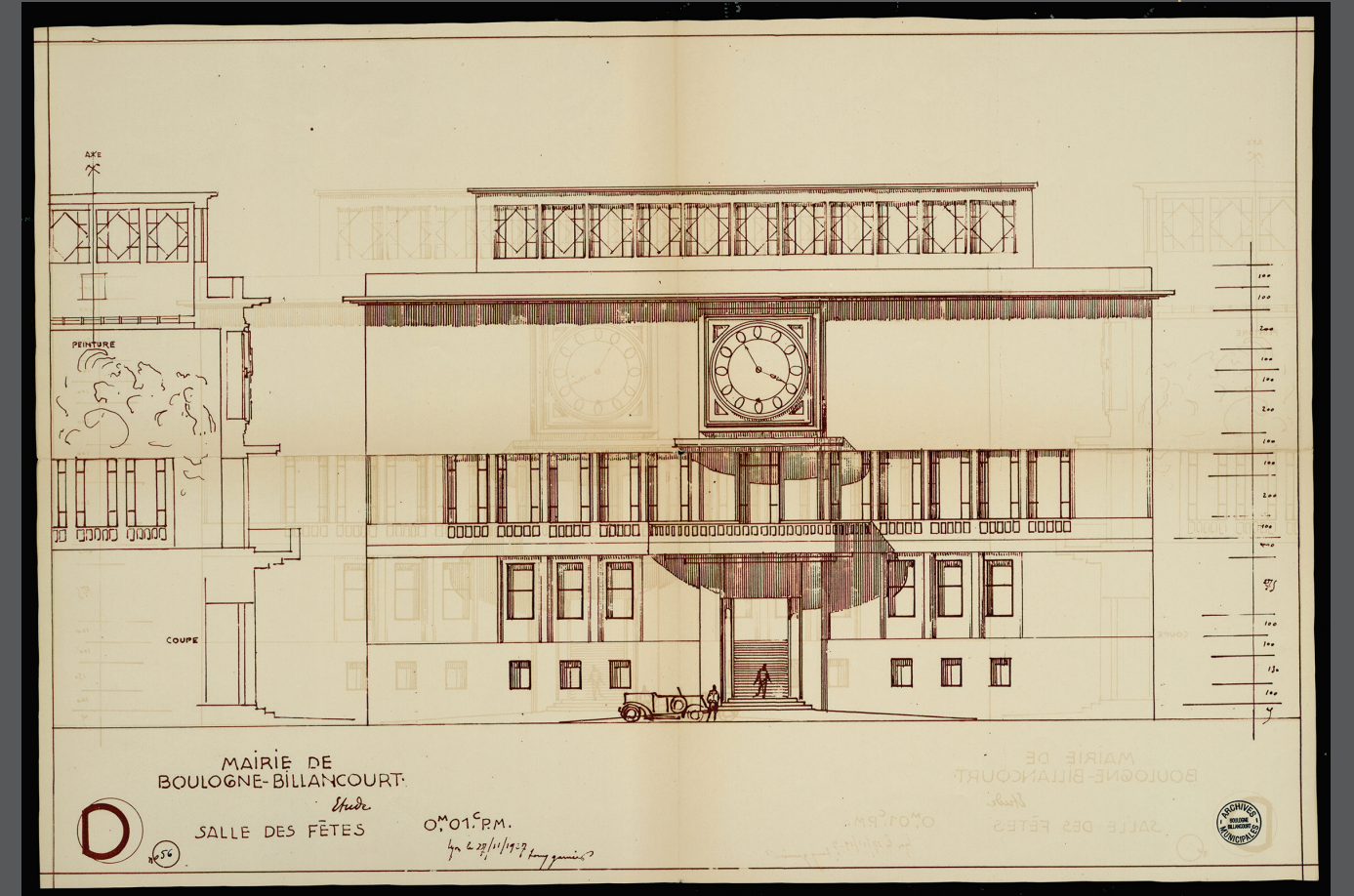
Projet de façade 27 novembre 1927 - 1 M1 56
