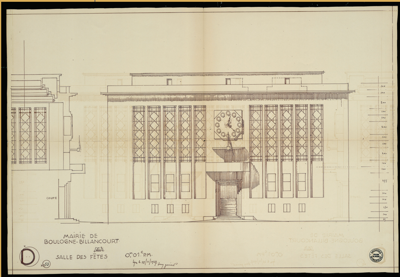
Projet de façade 28 novembre 1927 - 1 M1 53
