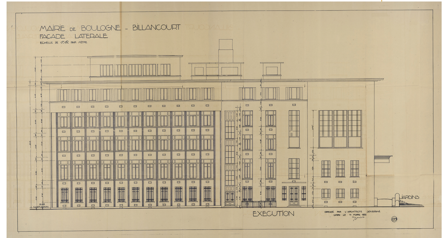
Plan d'exécution de la façade du bâtiment des réceptions 24 mars 1930 - 1 M3 122
