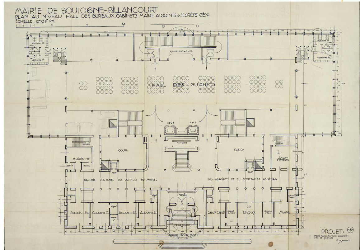
Plan du rez-de-chaussée 1 er octobre 1929- 1 M2 89
