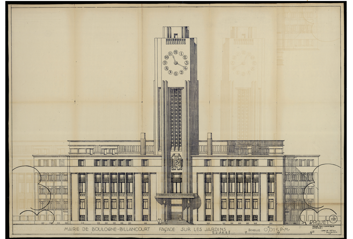
Projet de façade 1928 - 1 M2 75
