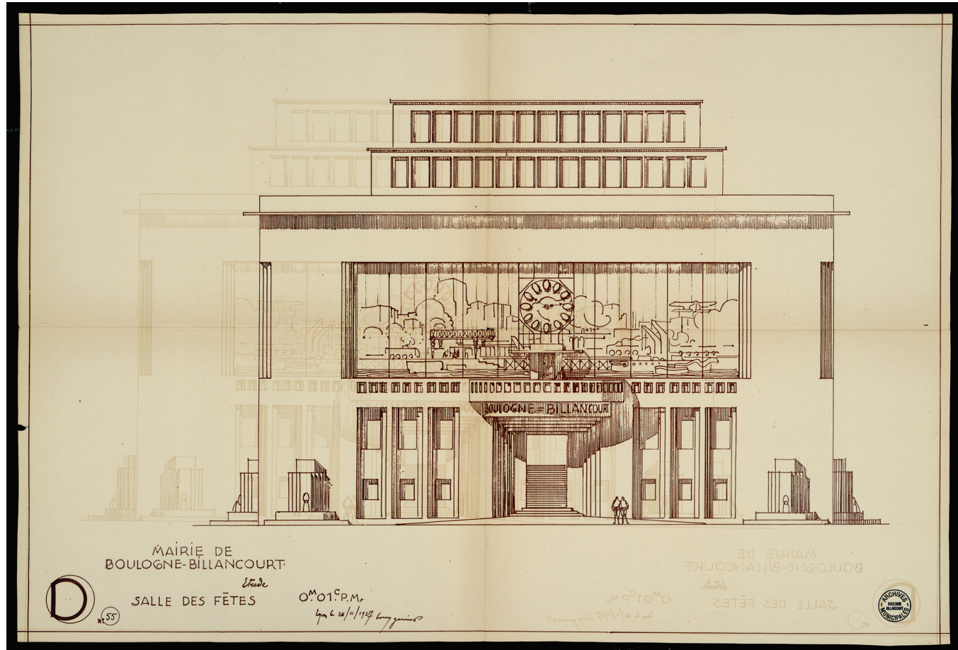
Projet de façade 26 novembre 1927 - 1 M1 55
