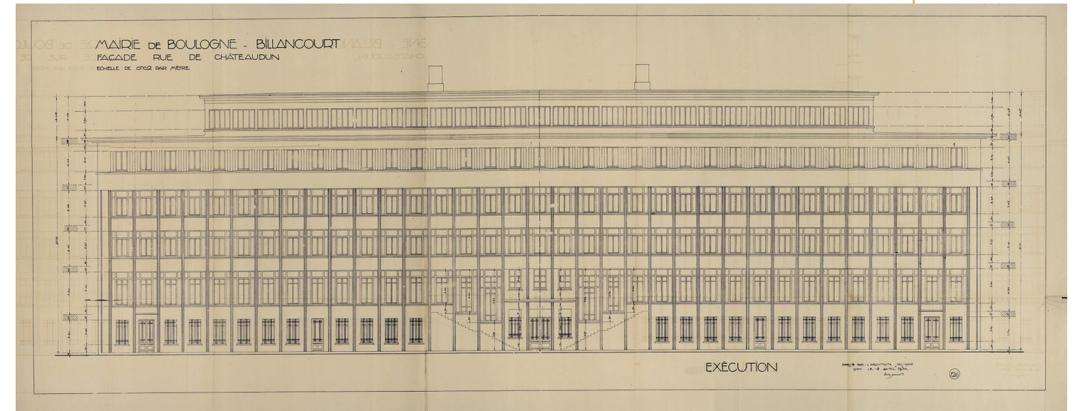
Plan d'exécution de la façade du bâtiment des services 1er octobre 1929 - 1 M3 126
