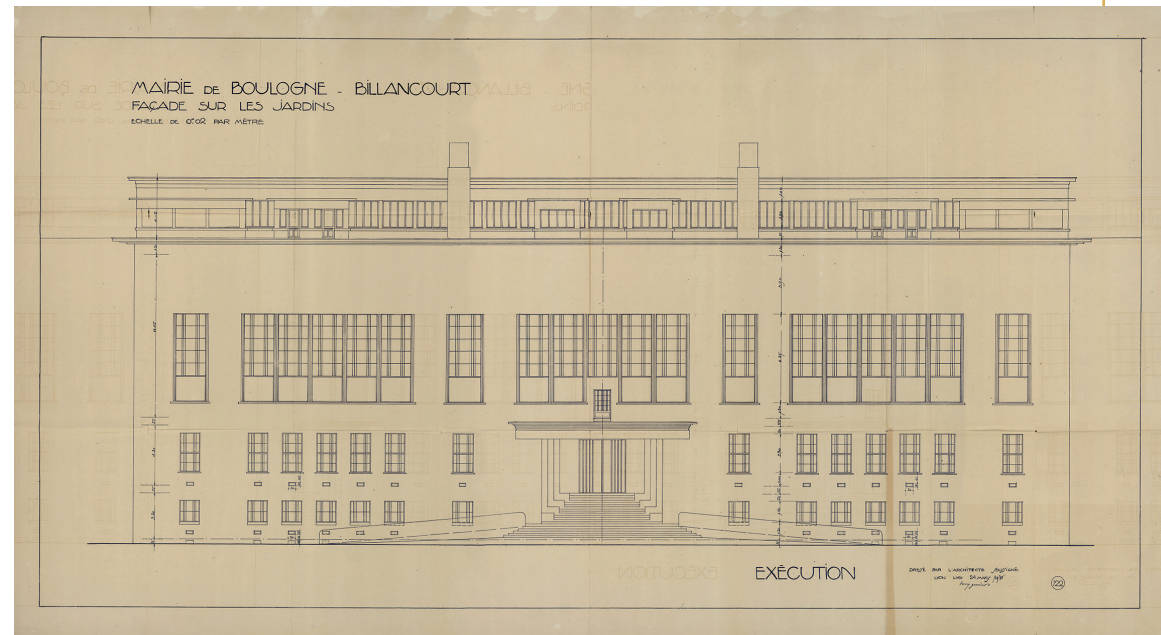
Plan d'exécution de la façade latérale 11 mars 1930 - 1 M3 123
